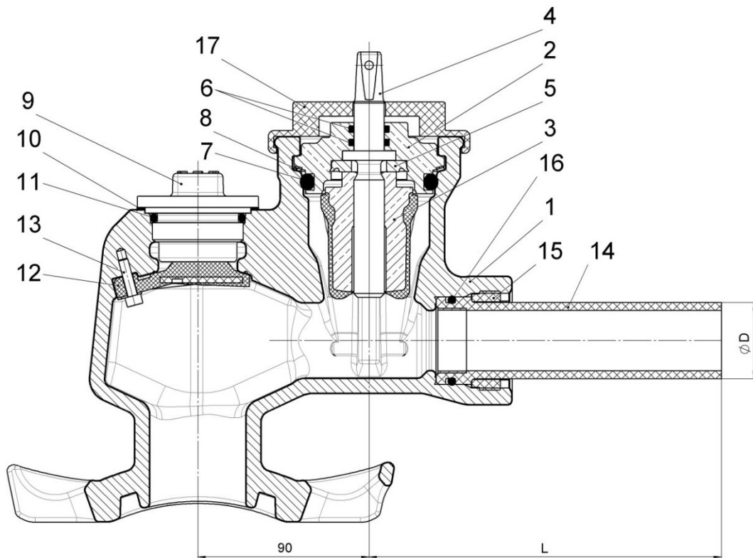
Abbildung: Anbohrarmatur Typ 1004 TOP PEHD
