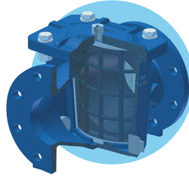
SCHNITTBILD
