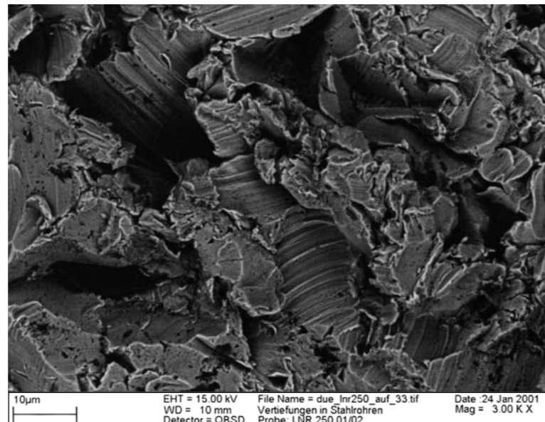
Abb. 3: Detailaufnahme einer mit Korund gestrahlten Stahloberfläche in etwa 3000-facher Vergrößerung (Rasterelektronenmikroskopaufnahme Fraunhofer-Institut ISC, Würzburg). Die Oberfläche ist durch den Strahlvorgang deutlich zerklüftet und erodiert. Sie bietet dem nachfolgenden Emaillierprozess eine ideale Voraussetzung für den Aufbau des Werkstoffverbundes.
