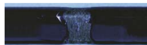
Dehnungsinduziertes Versagensbild des Emails im Biegeversuch im Bereich der plastischen Verformung (Krafteinleitung). Außerhalb der plastischen Zone, links und rechts, schadensfreie Emaillierung.
