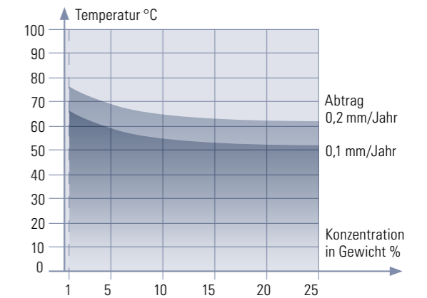
Korrosionsgeschwindigkeit in NaOH-wässrigen Lösungen
