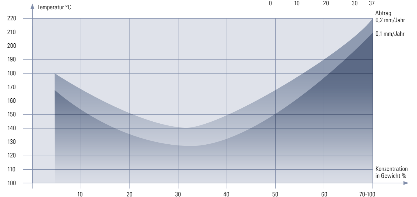
Korrosionsgeschwindigkeit in H 2 SO 4 -wässrigen Lösungen
