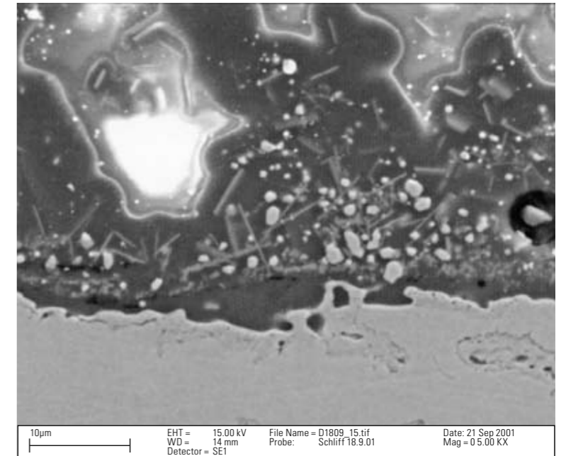
Abb. 2: Detailaufnahme einer Verbundschicht Email (hier mit Gusseisen GGG Rasterelektronenmikroskopaufnahme Fraunhofer-Institut ISC, Würzburg) in etwa 5000-facher Vergrößerung. Deutlich sichtbar die (Mikro-) Rauigkeit der Oberfläche (hell, unten) mit Hinterschneidungen. Nach oben anschließend ein dünner homogener erscheinender Saum von etwa 2 µm Dicke, weiter anschließend die eigentliche Verbundschicht von deutlich über 10 µm Dicke mit unterschiedlichen Ausscheidungen (i.W. Eisentitanatkristalle in Nadel- bzw. Plättchenform) und Einlagerungen.
