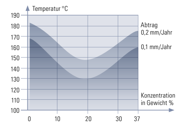
Korrosionsgeschwindigkeit in HCl-wässrigen Lösungen
