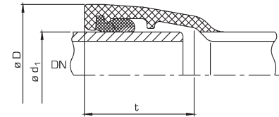
Muffe für Formstücke
